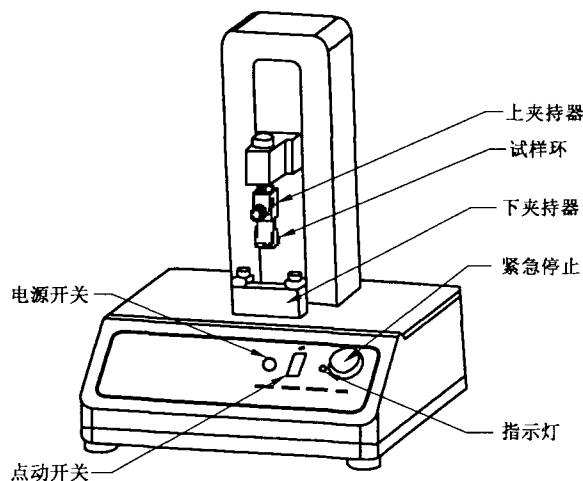
图 5 自动环形初粘性能试验机示意图
