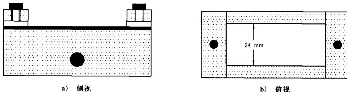
图1 试验夹具示意图
