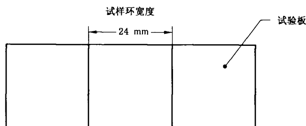
图 3 试样环在试验板上的接触位置
