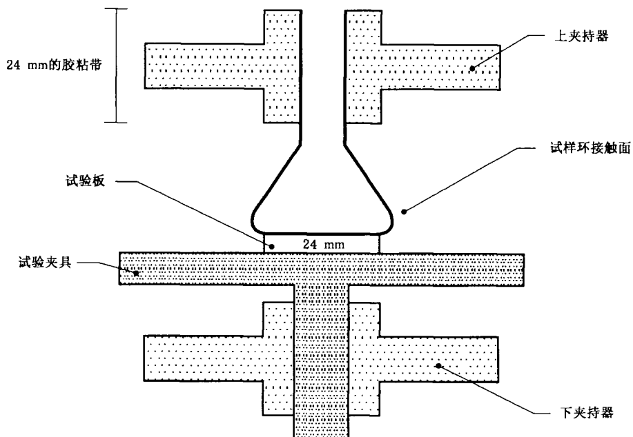
图 2 试样环测试示意图
